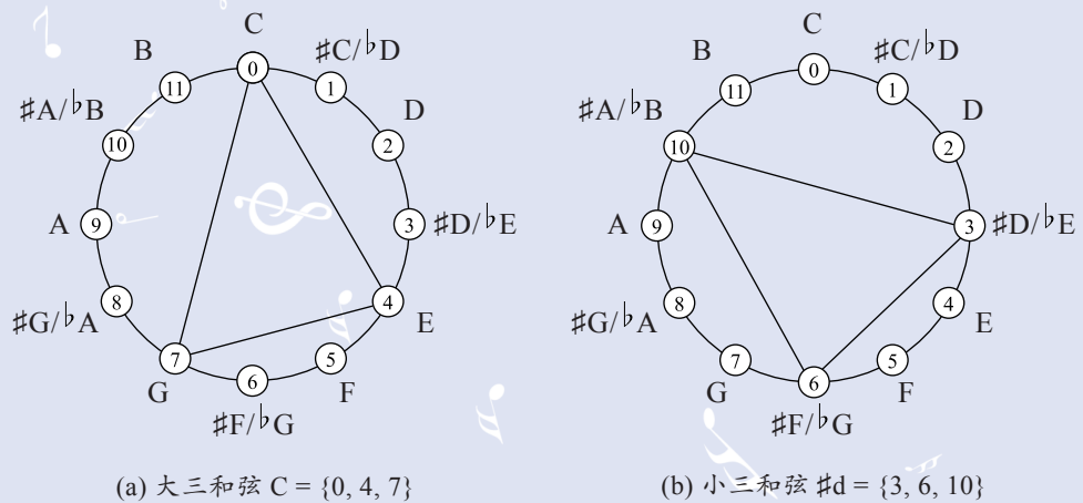
图 1. 音类圆周上的三和弦
