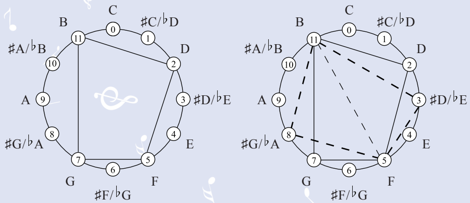
(a) 属七和弦 G — B — D — F
