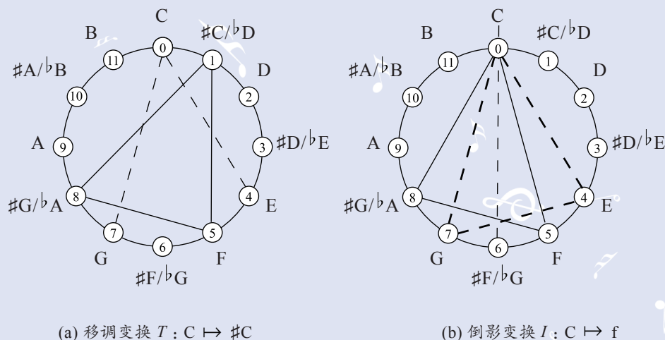
图 2. 群 \mathcal{D} 在大、小三和弦上的作用
